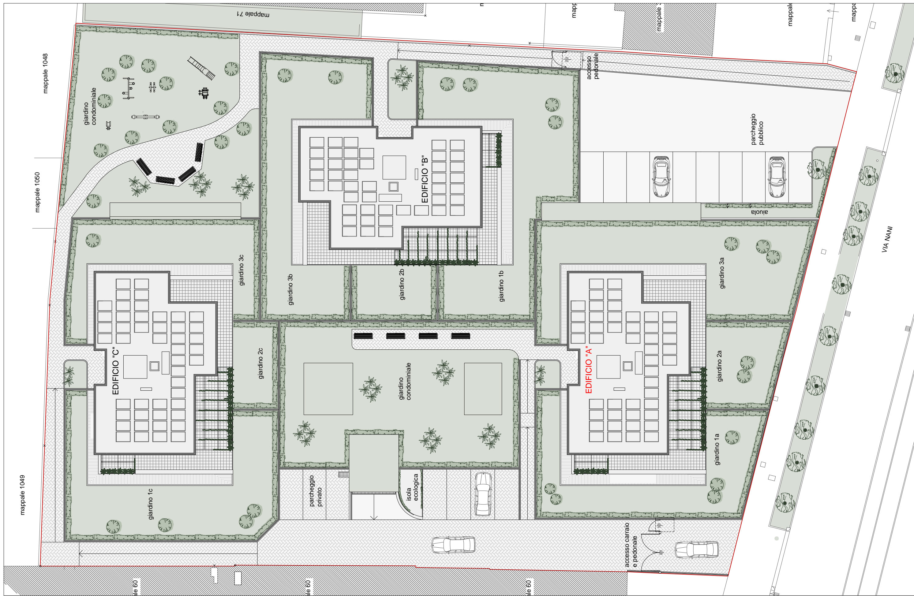
PLANIMETRIA DI INTERVENTO _ FUORI SCALA
