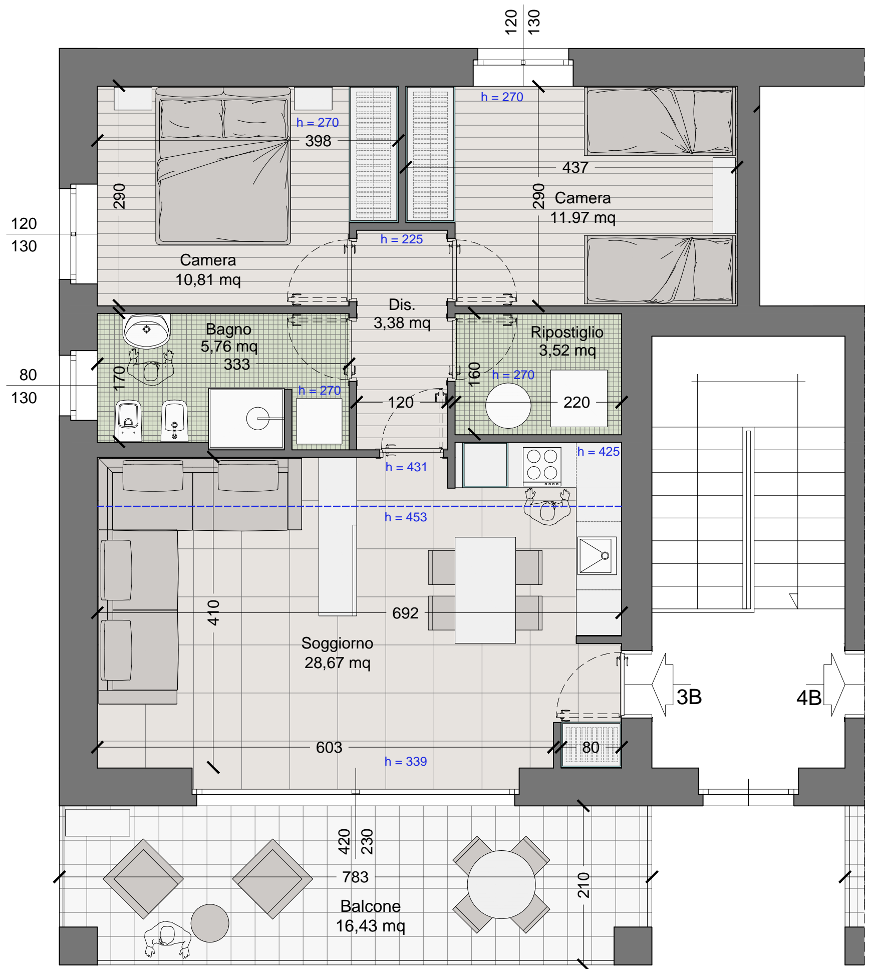
scala 1:50
