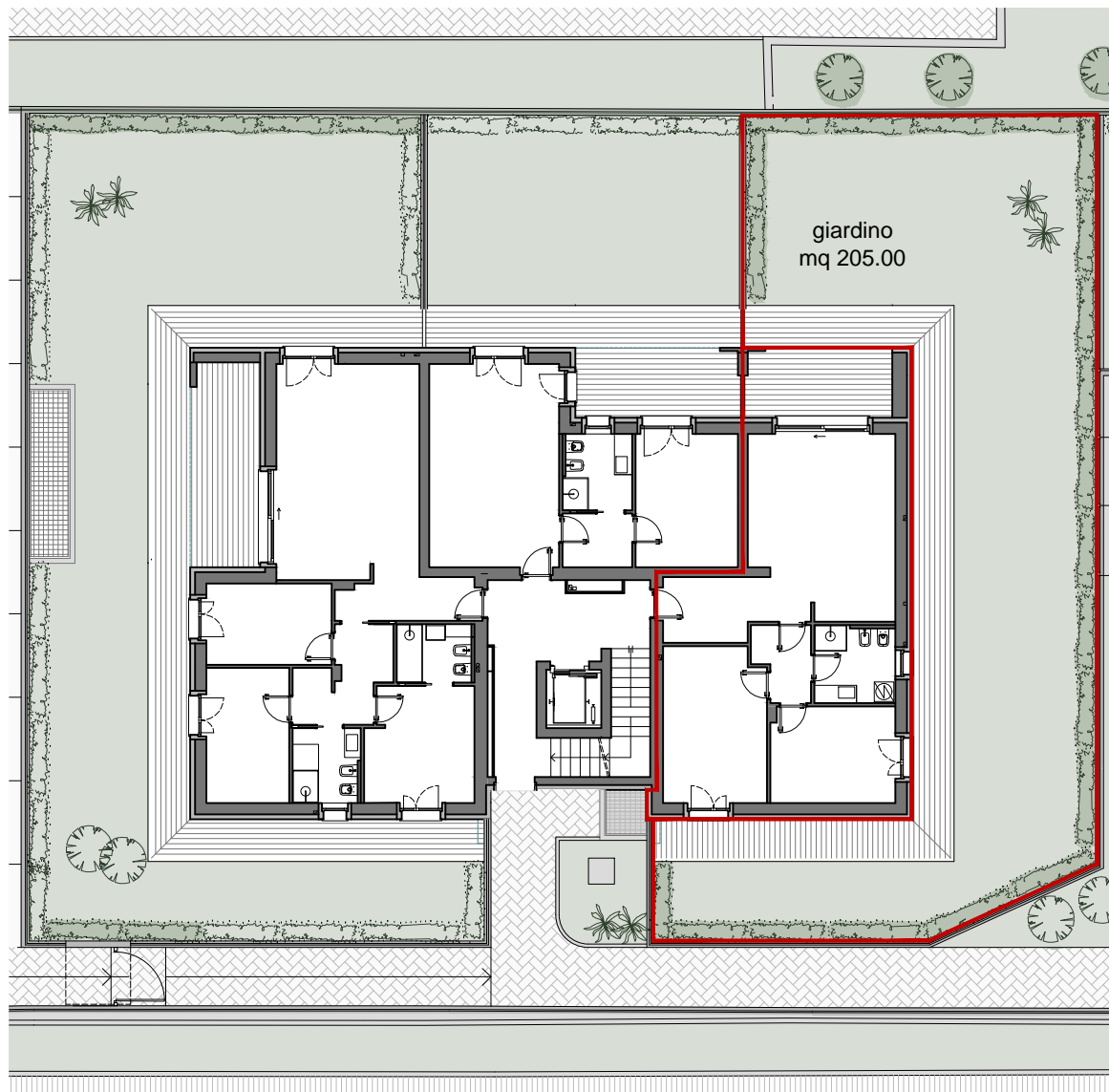
EDIFICIO A - PIANO TERRA - APPARTAMENTO 3a
