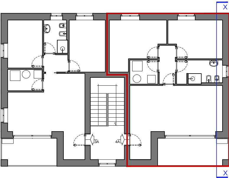
PIANTA - SEZIONE CON INDICAZIONE ALTEZZE _ FUORI SCALA
