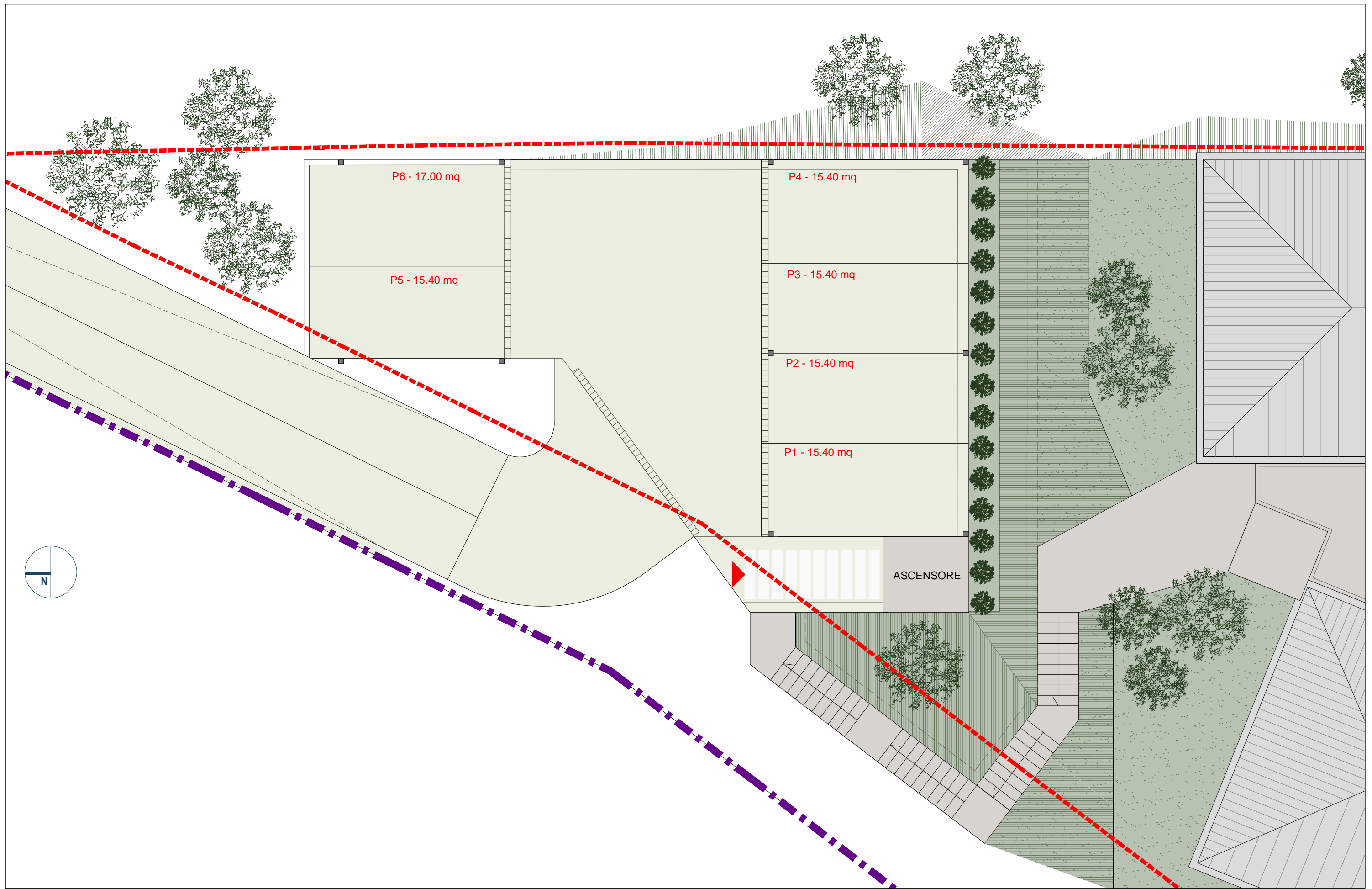
PLANIMETRIA POSTI AUTO
