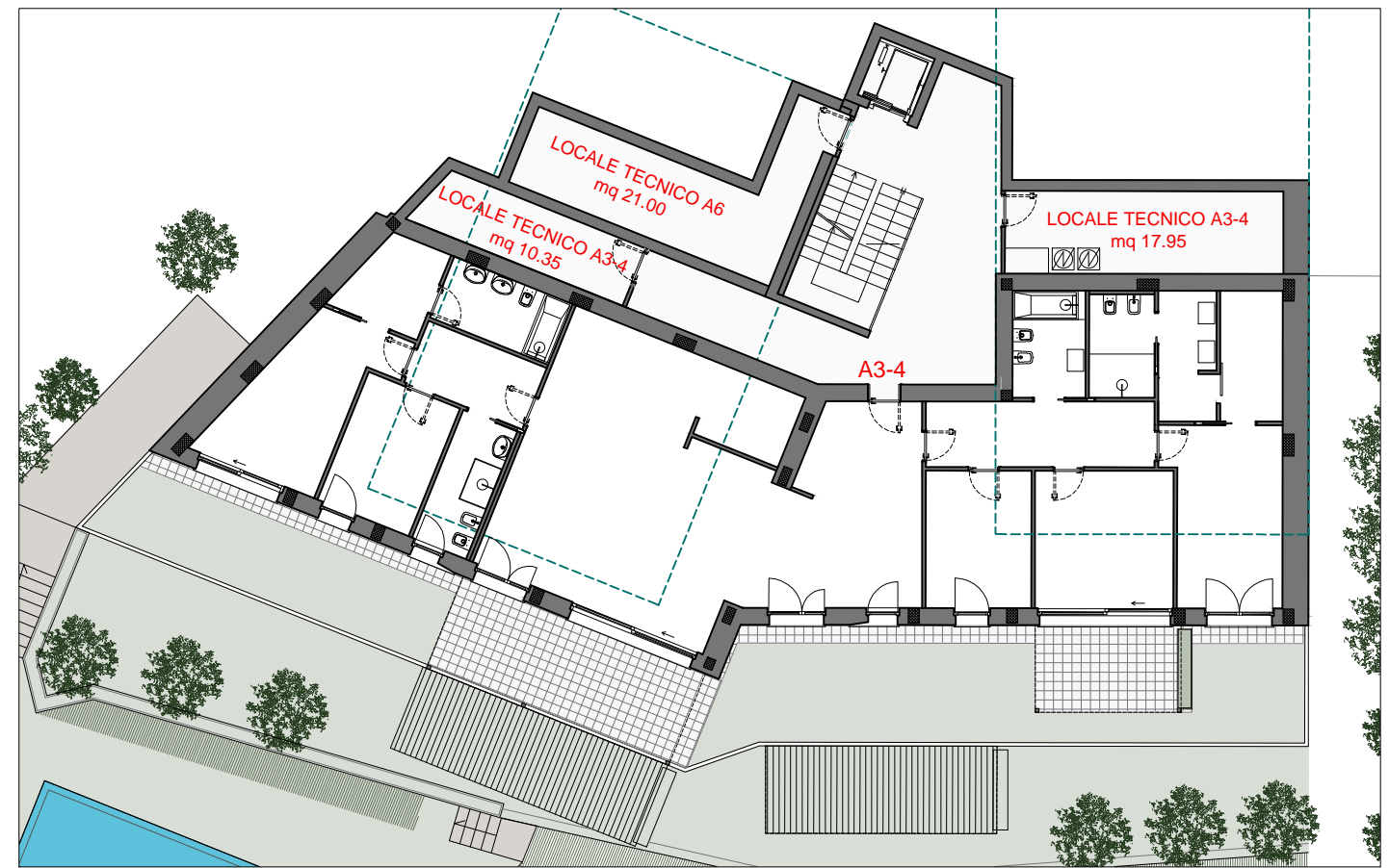
PIANTA QUOTA 302.65
