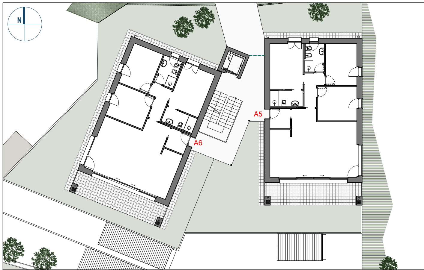
PIANTA QUOTA 306.30
