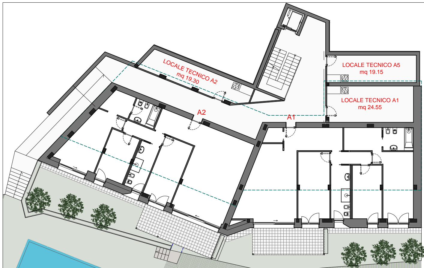
PIANTA QUOTA 299.00
