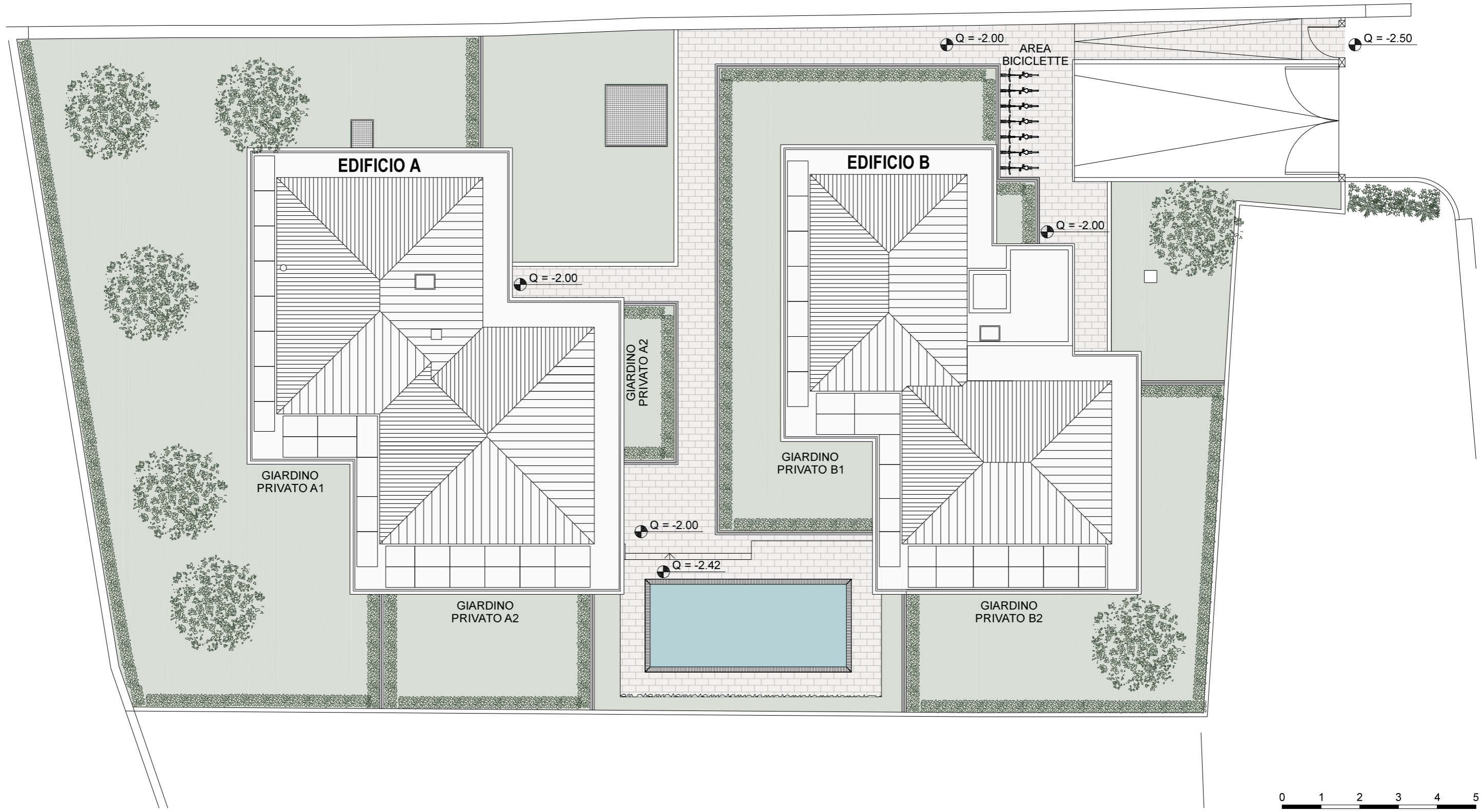
PLANIMETRIA GENERALE
