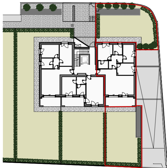
EDIFICIO C - PIANO TERRA - APPARTAMENTO C1
