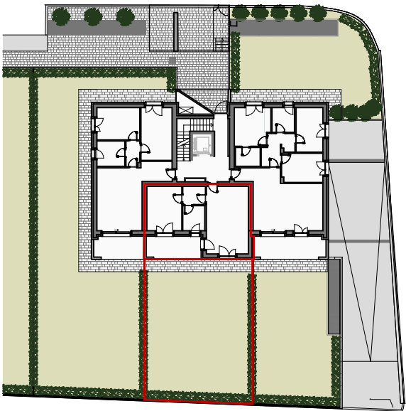
EDIFICIO C - PIANO TERRA - APPARTAMENTO C2
