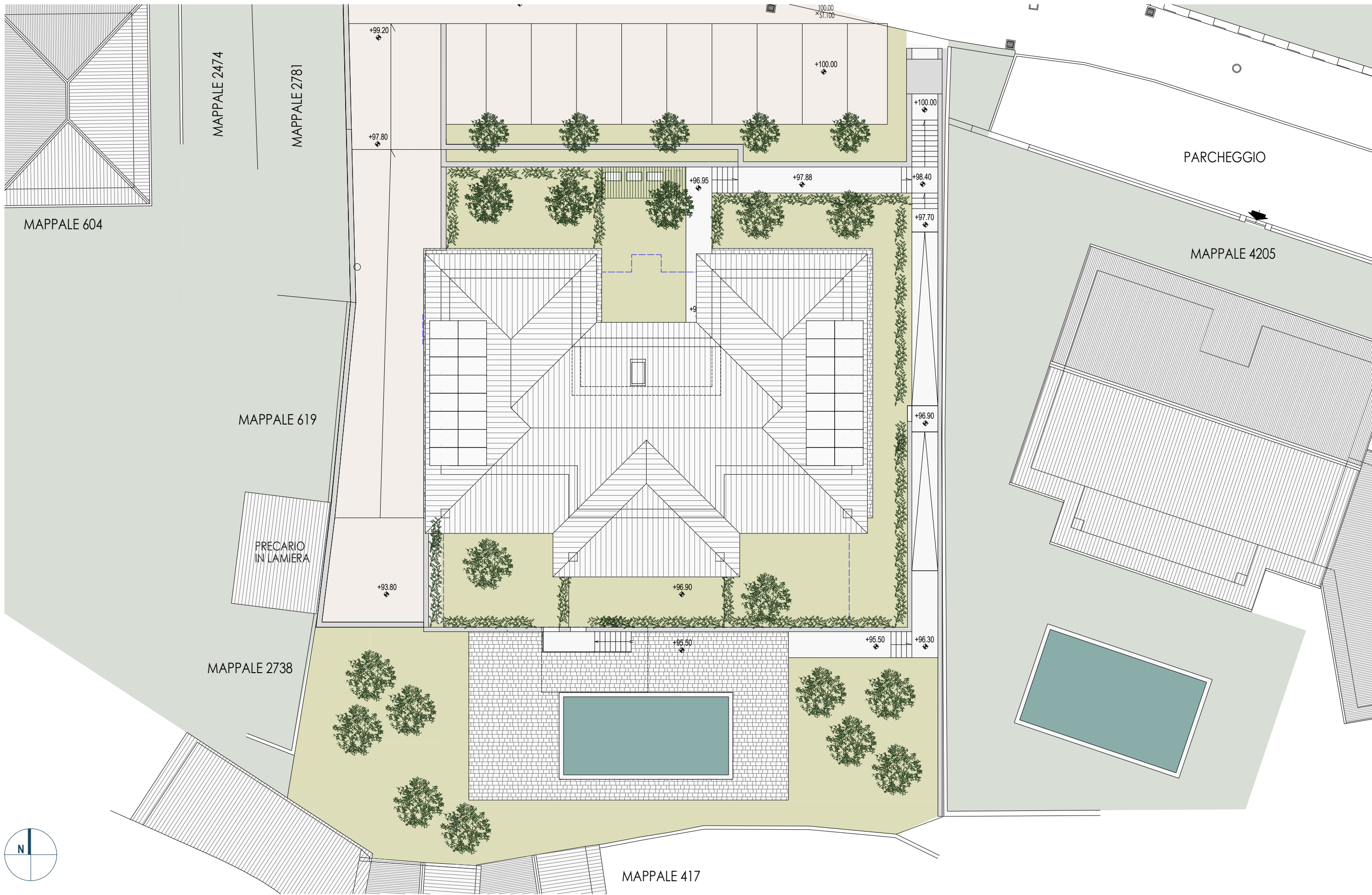
PLANIMETRIA GENERALE
