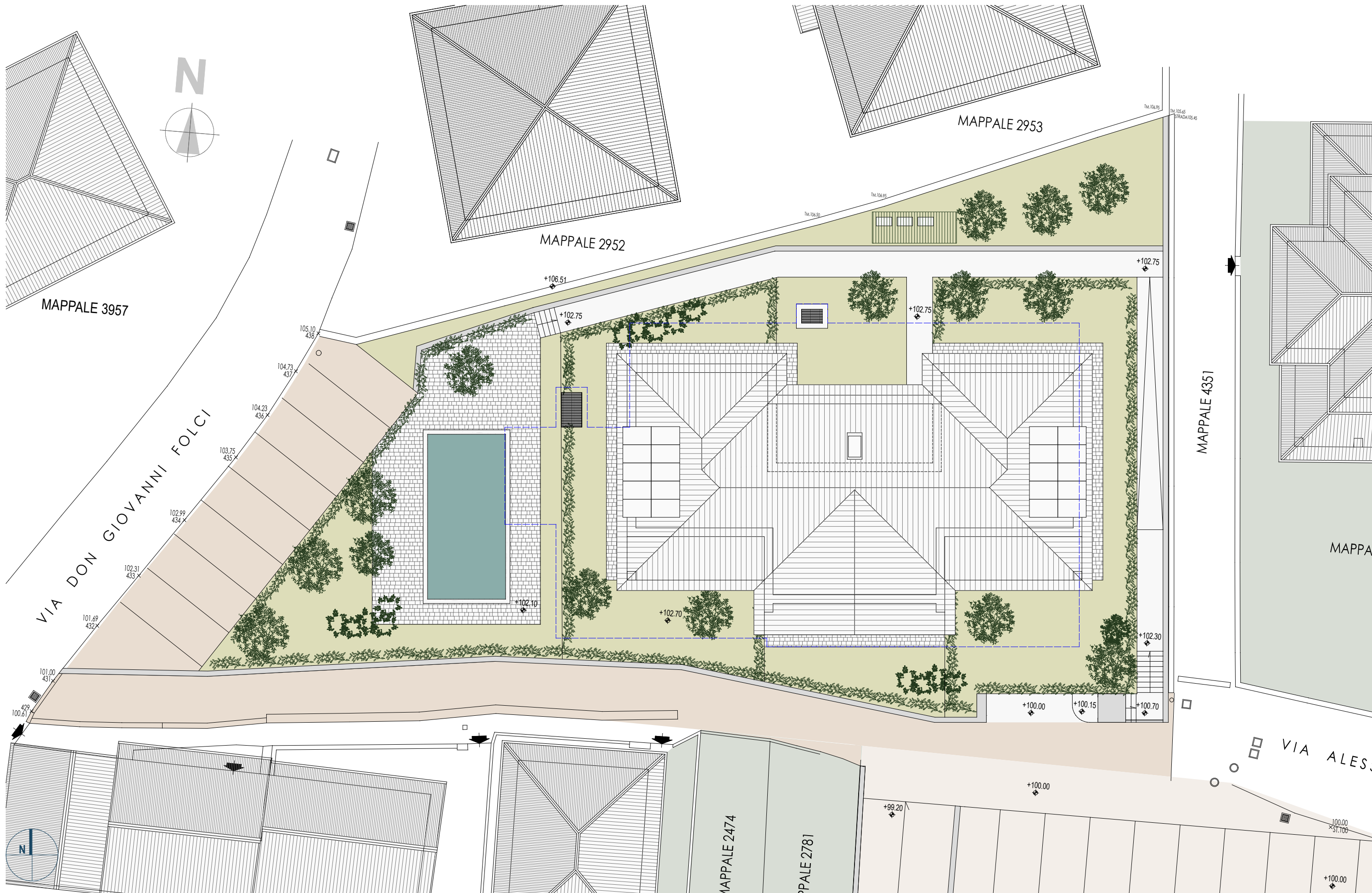
PLANIMETRIA GENERALE
